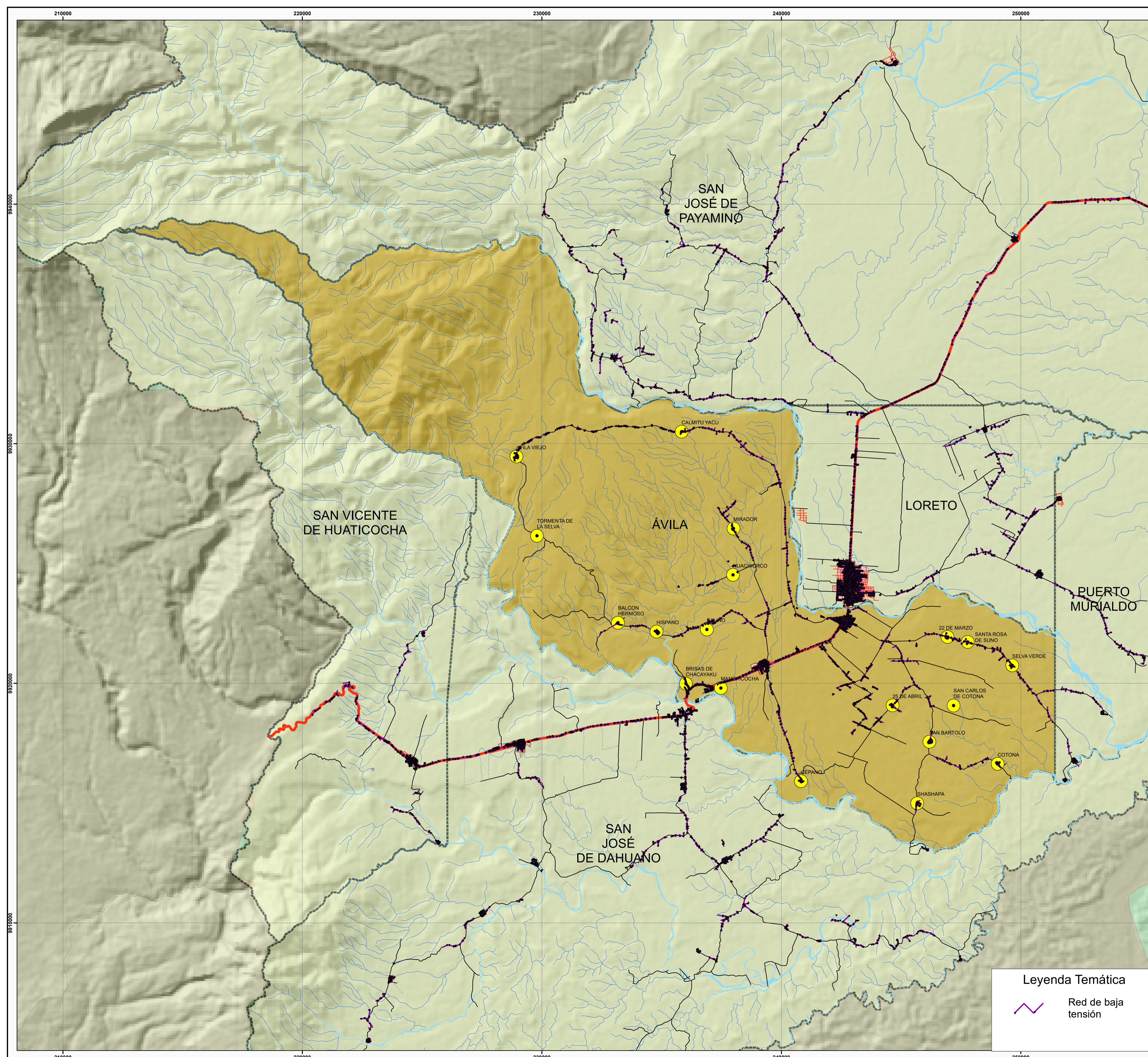
14.2 - Mapa de redes eléctricas (baja tensión) de la parroquia de Ávila Huiruno
